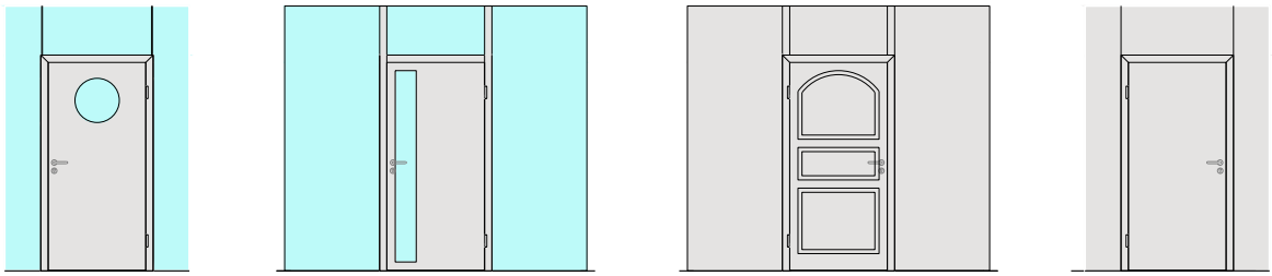
Einbau in FeuerschutzTeam Festverglasung mit Glasleisten geschraubt, Türe gefälzt
