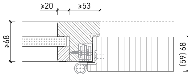
Einbau in FeuerschutzTeam Festverglasung mit Glasleisten geschraubt, Türe gefälzt
