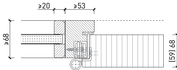
Einbau in FeuerschutzTeam Festverglasung mit angefrästen Glasleisten, Türe gefälzt
