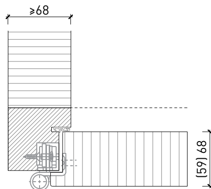
Einbau in FeuerschutzTeam Vollwand, Türe gefälzt
